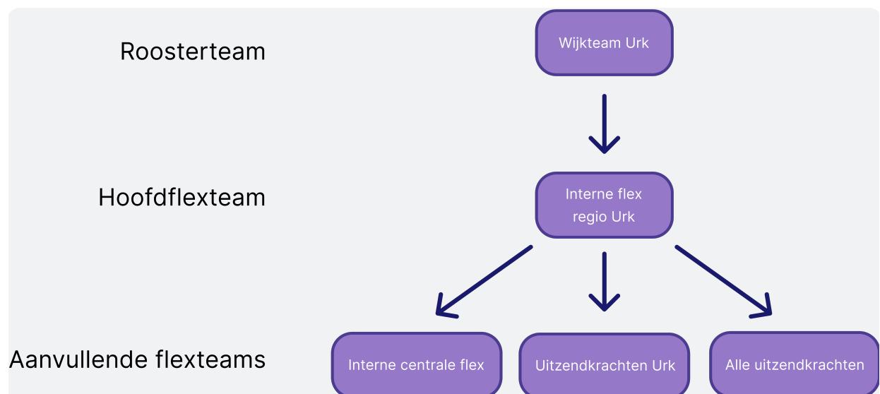
Afbeelding 2: Inrichtingsvoorbeeld met decentrale flexpool als hoofdflexteam
